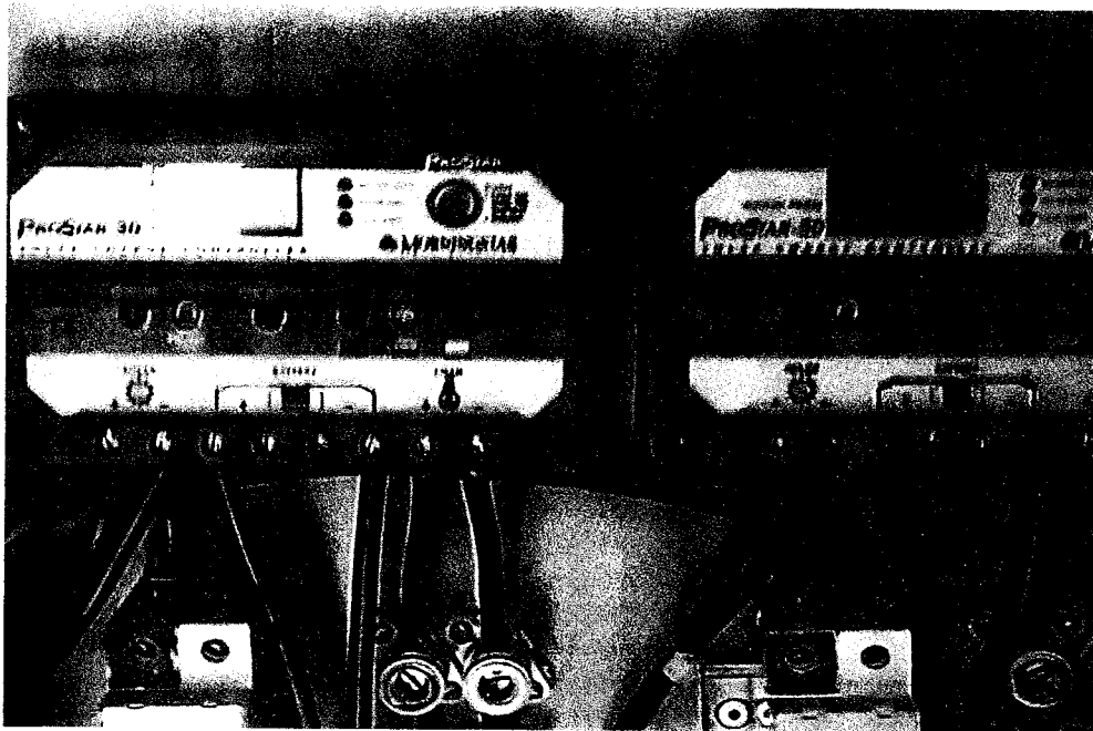
Gruppo regolatori di tensione (rif foto a seguito fornitura nel 2012)
